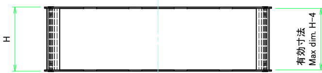
Wパネル1 / W Panel 1
