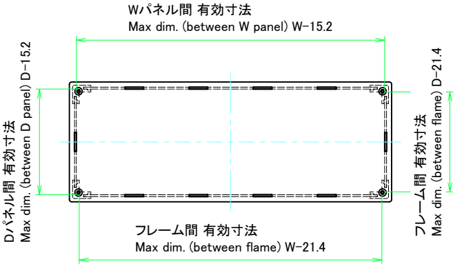
下カバー / Bottom cover
